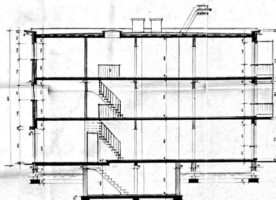
DOORSNEDE A-B
